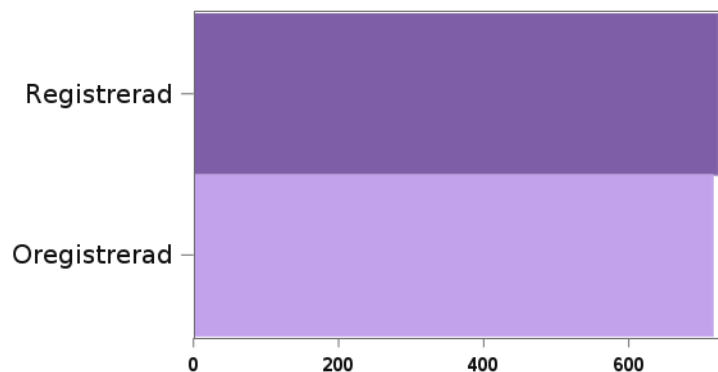
Diagram 12: Total Mortalitet för Registrerade och Oregistrerade - Rottweiler 2016-2021
